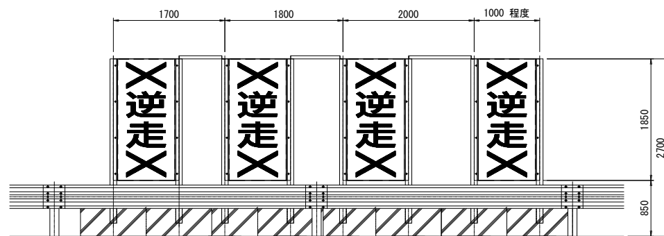
立面図（道路より）
