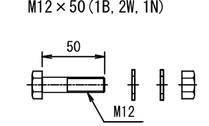
ブラケット接続ボルト
