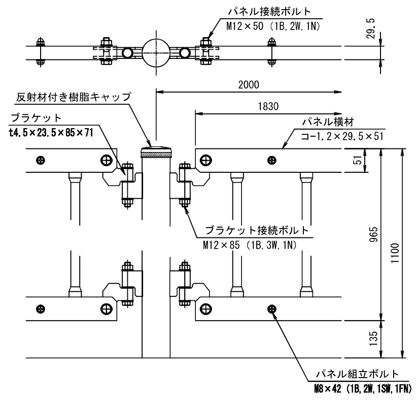
接合部拡大図
