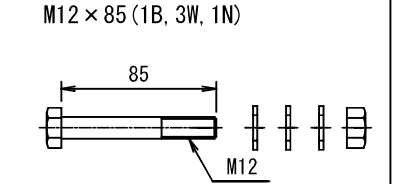
ブラケット接続ボルト
