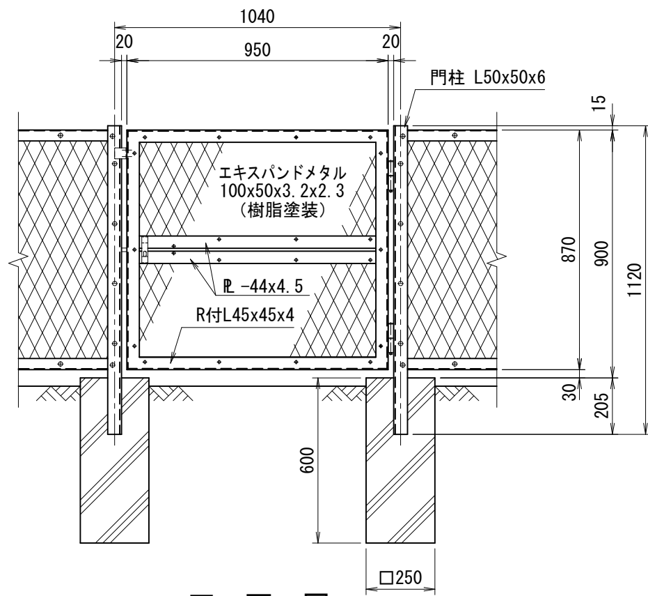
正面図 (S=1/20)
