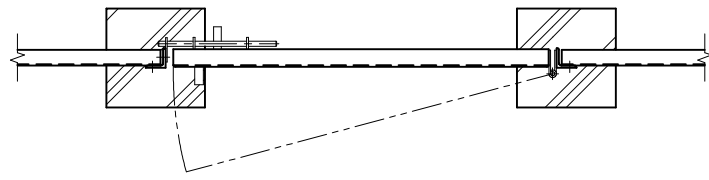
平面図 (S=1/20)
