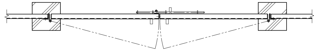
平面図 (S=1/20)
