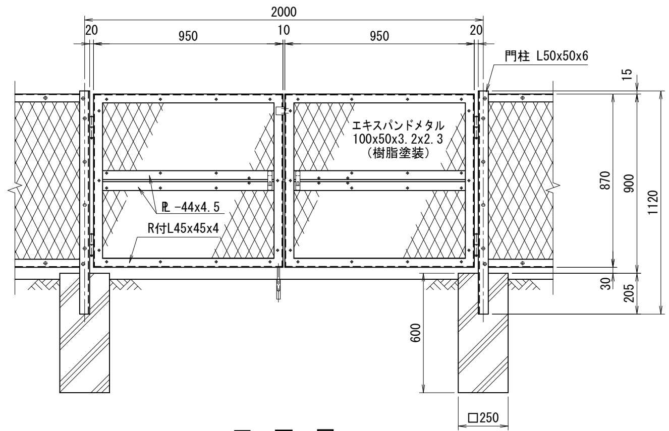
正面図 (S=1/20)
