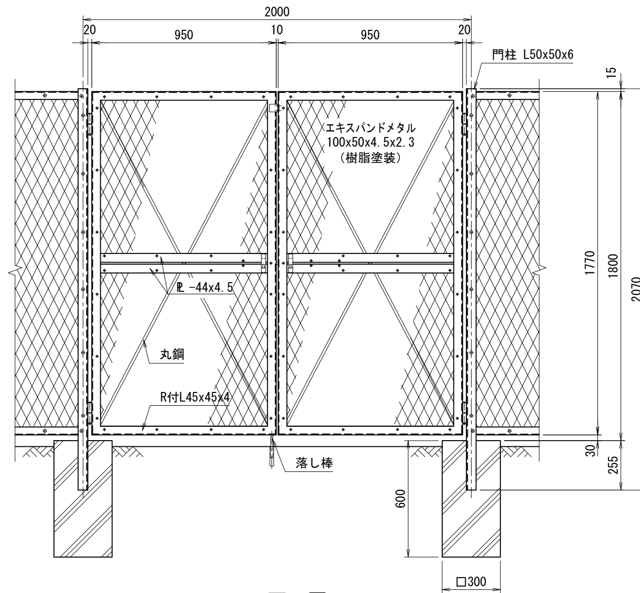
正面図 (S=1/20)
