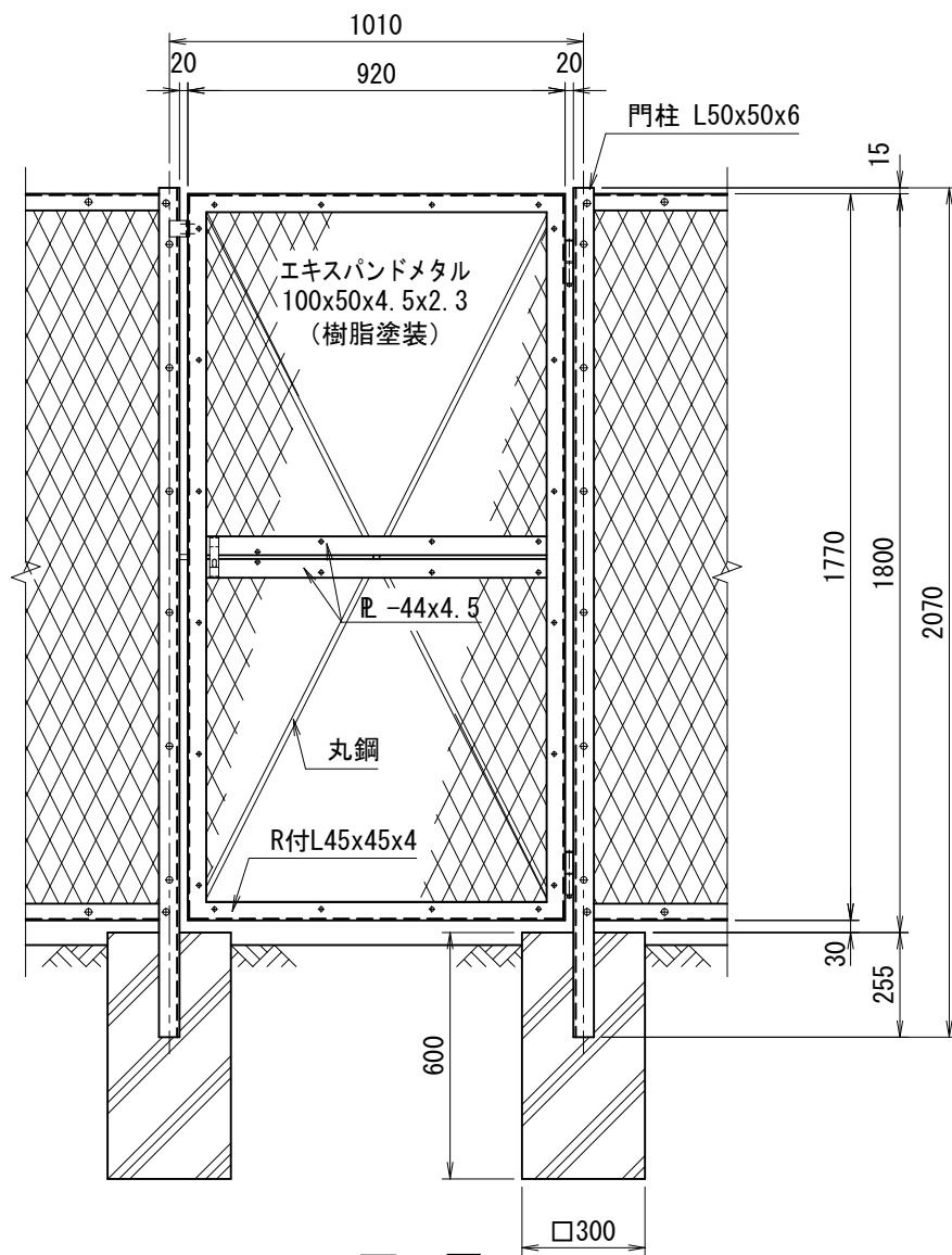
正面図 (S=1/20)
