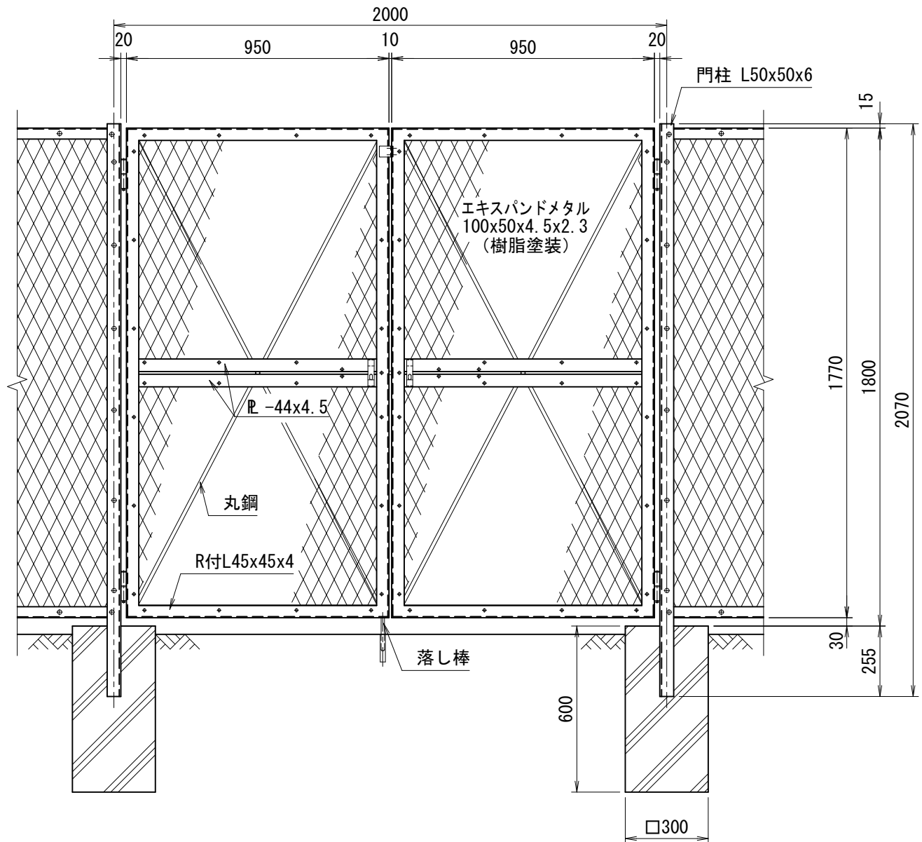
正面図 (S=1/20)
