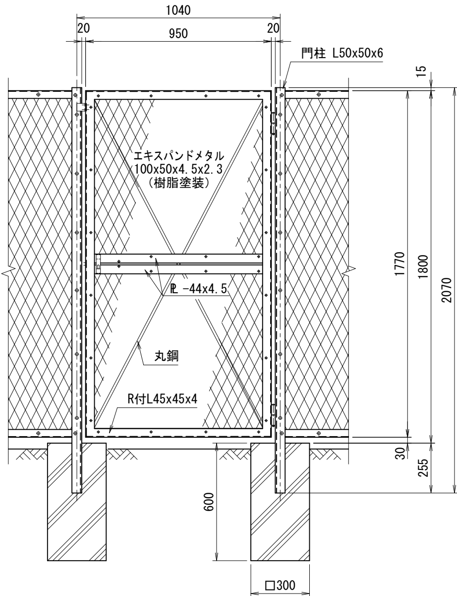
正面図 (S=1/20)
