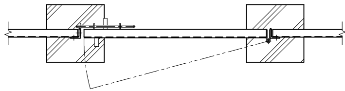
平面図 (S=1/20)
