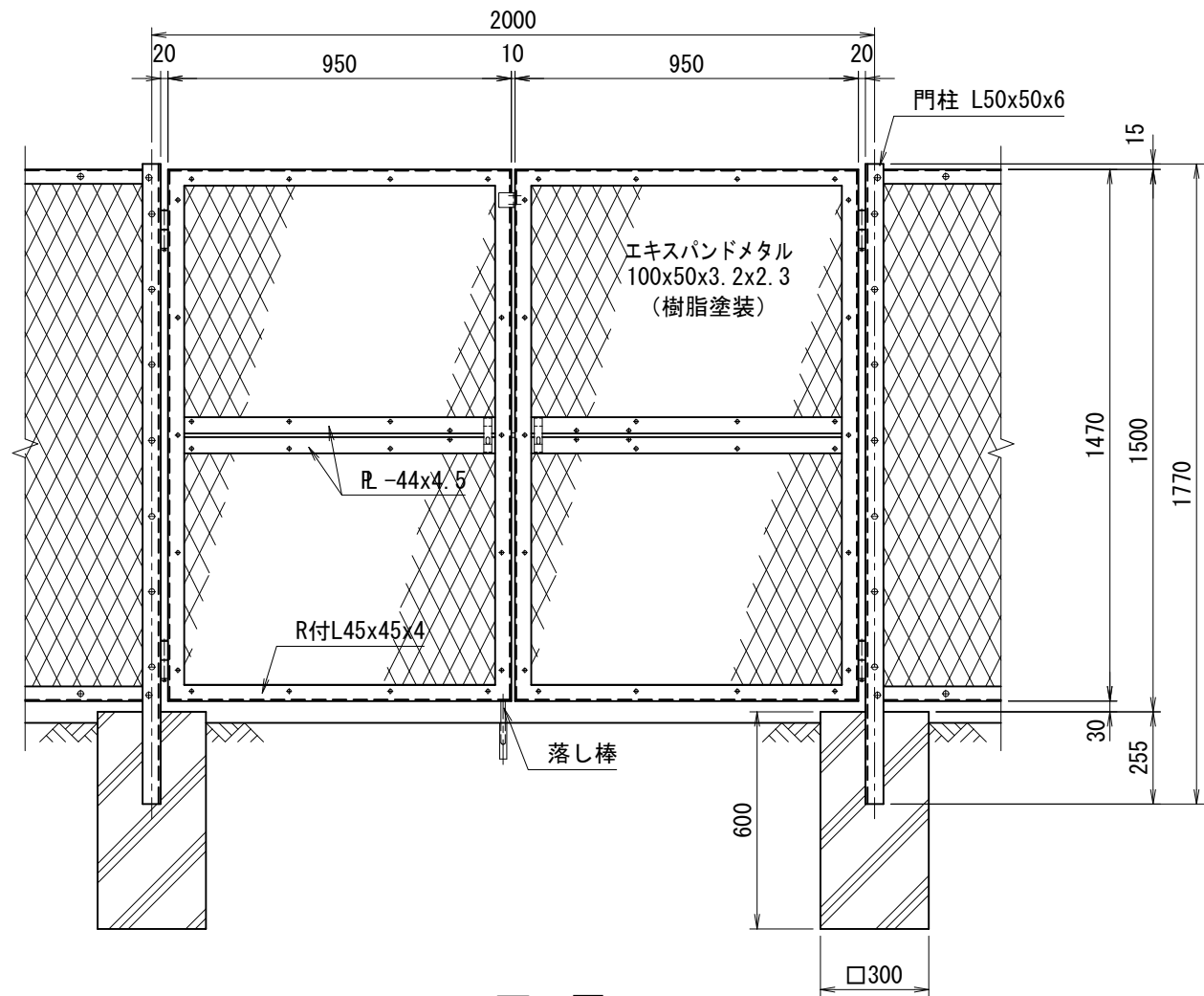
正面図 (S=1/20)
