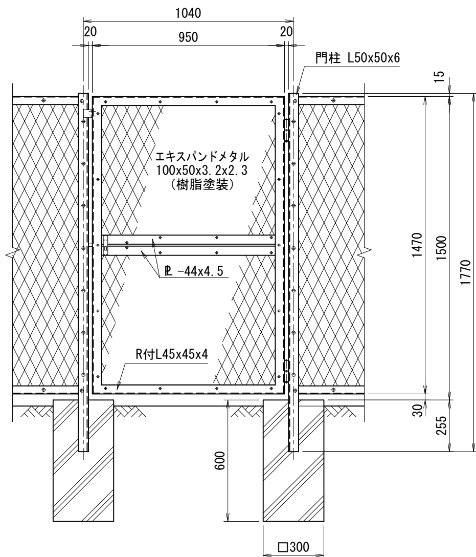
正面図 (S=1/20)
