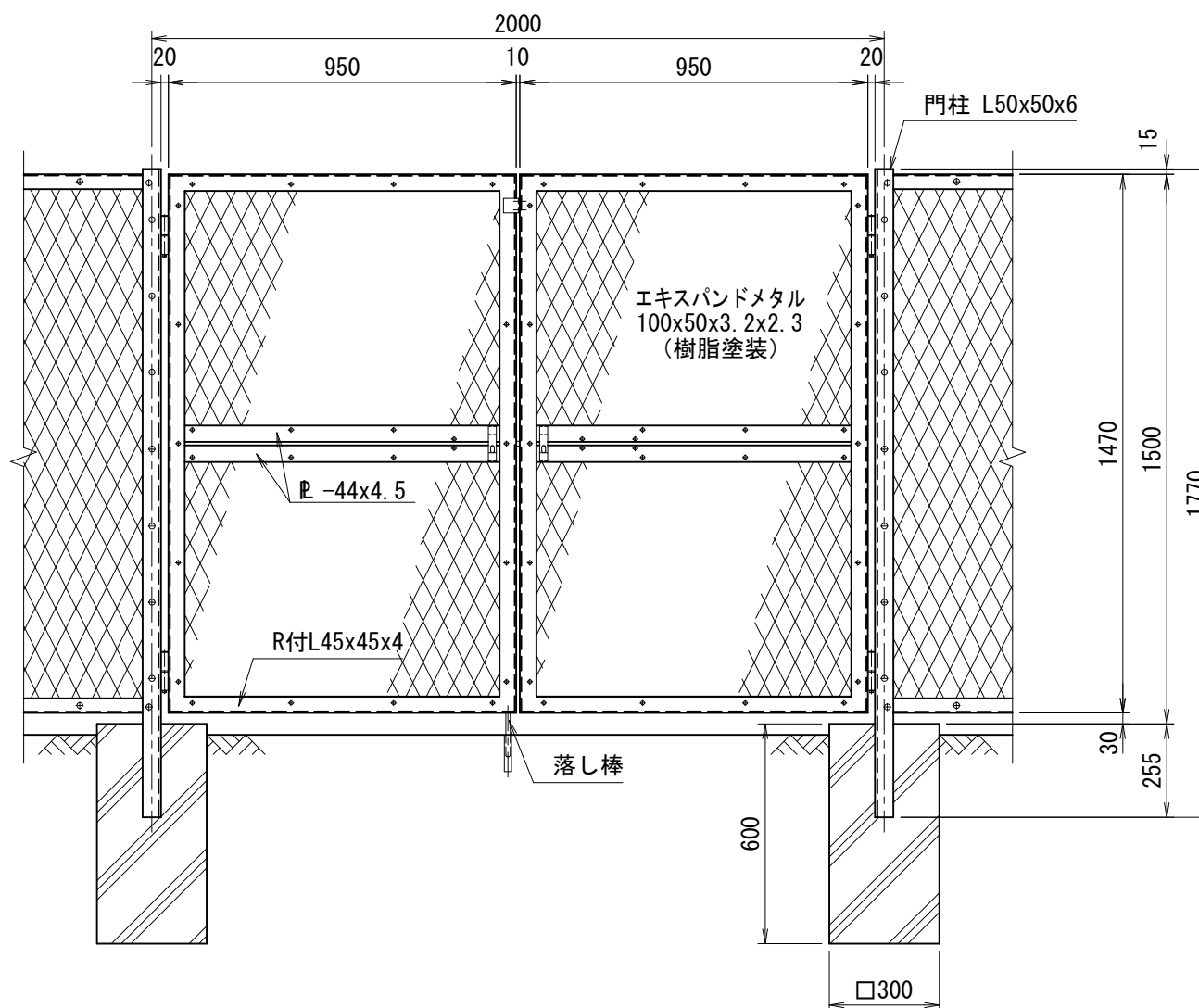
正面図 (S=1/20)
