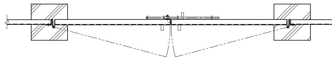
平面図 (S=1/20)
