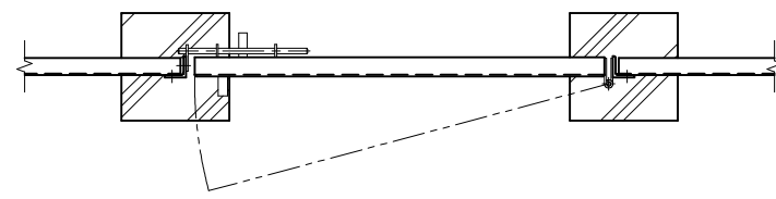
平面図 (S=1/20)
