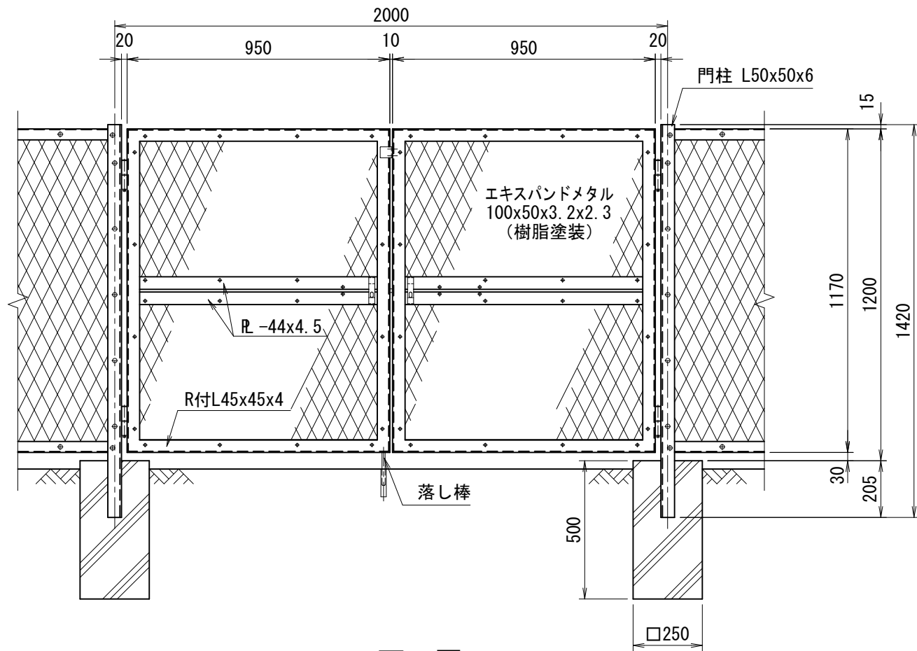
正面図 (S=1/20)
