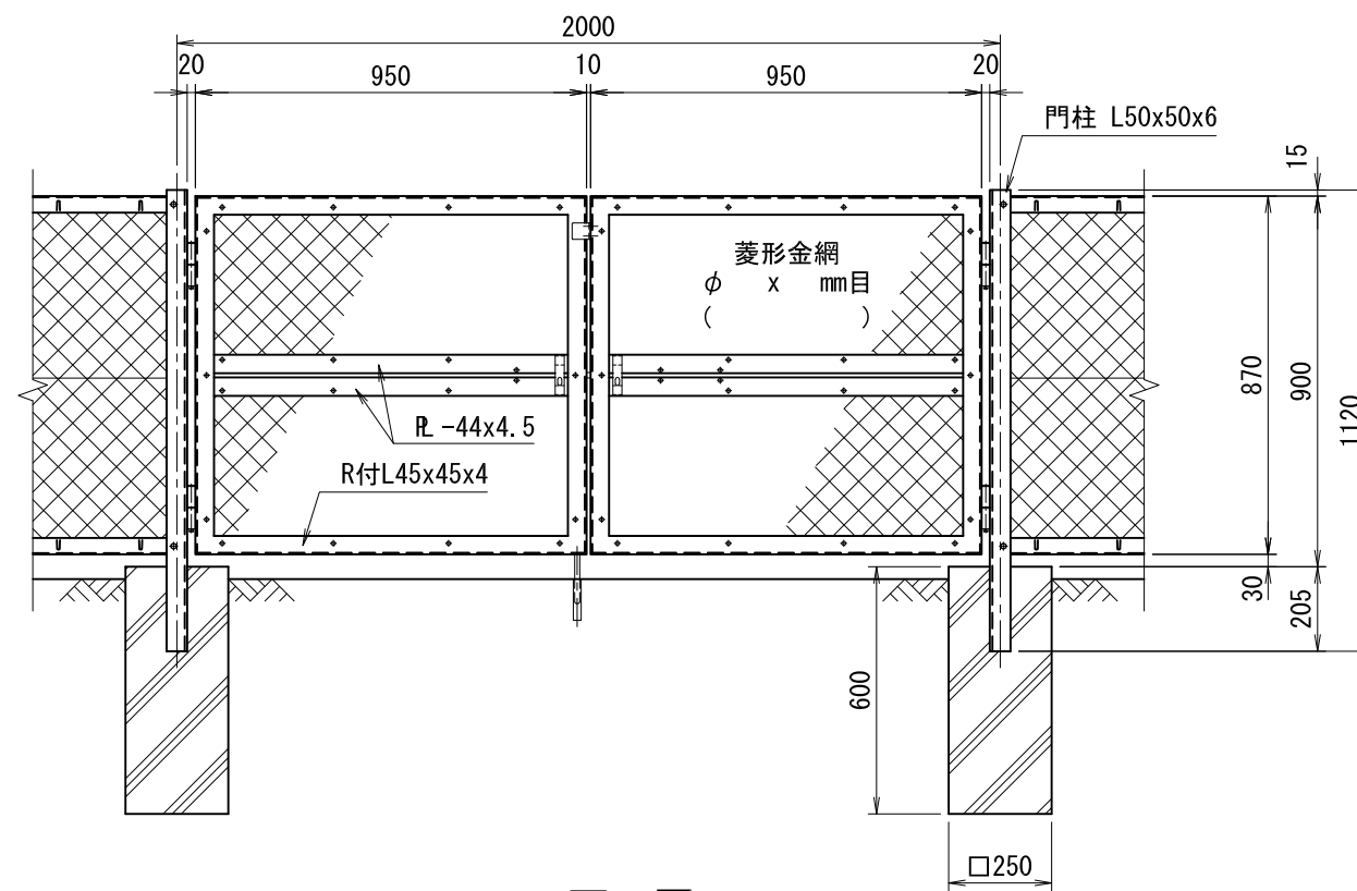
正面図 (S=1/20)
