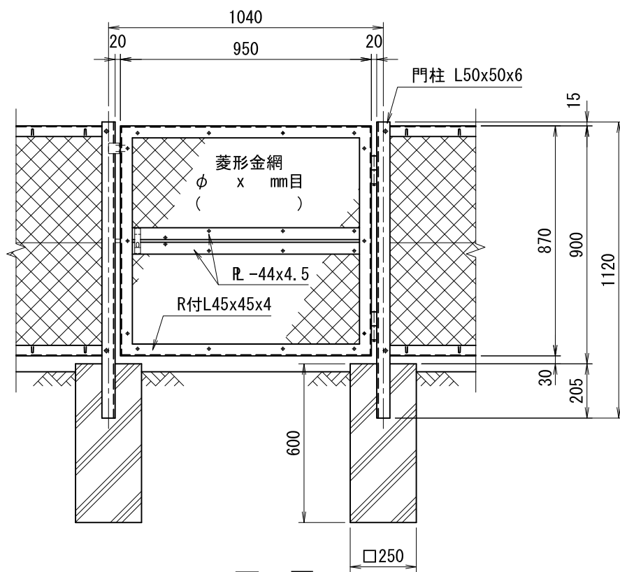
正面図 (S=1/20)
