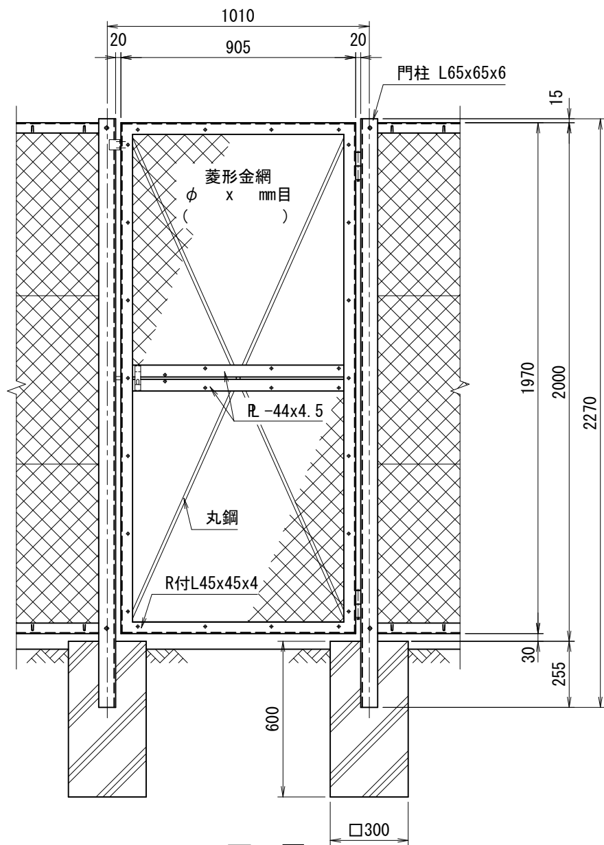
正面図 (S=1/20)
