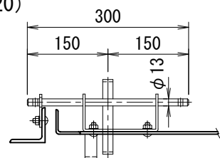
正面図 (S=1/20)
