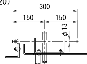
正面図 (S=1/20)
