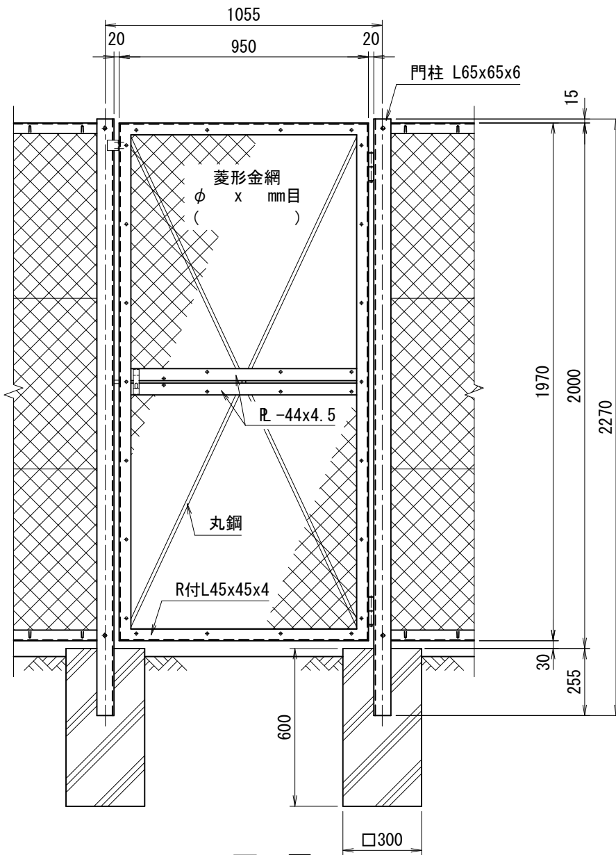
正面図 (S=1/20)
