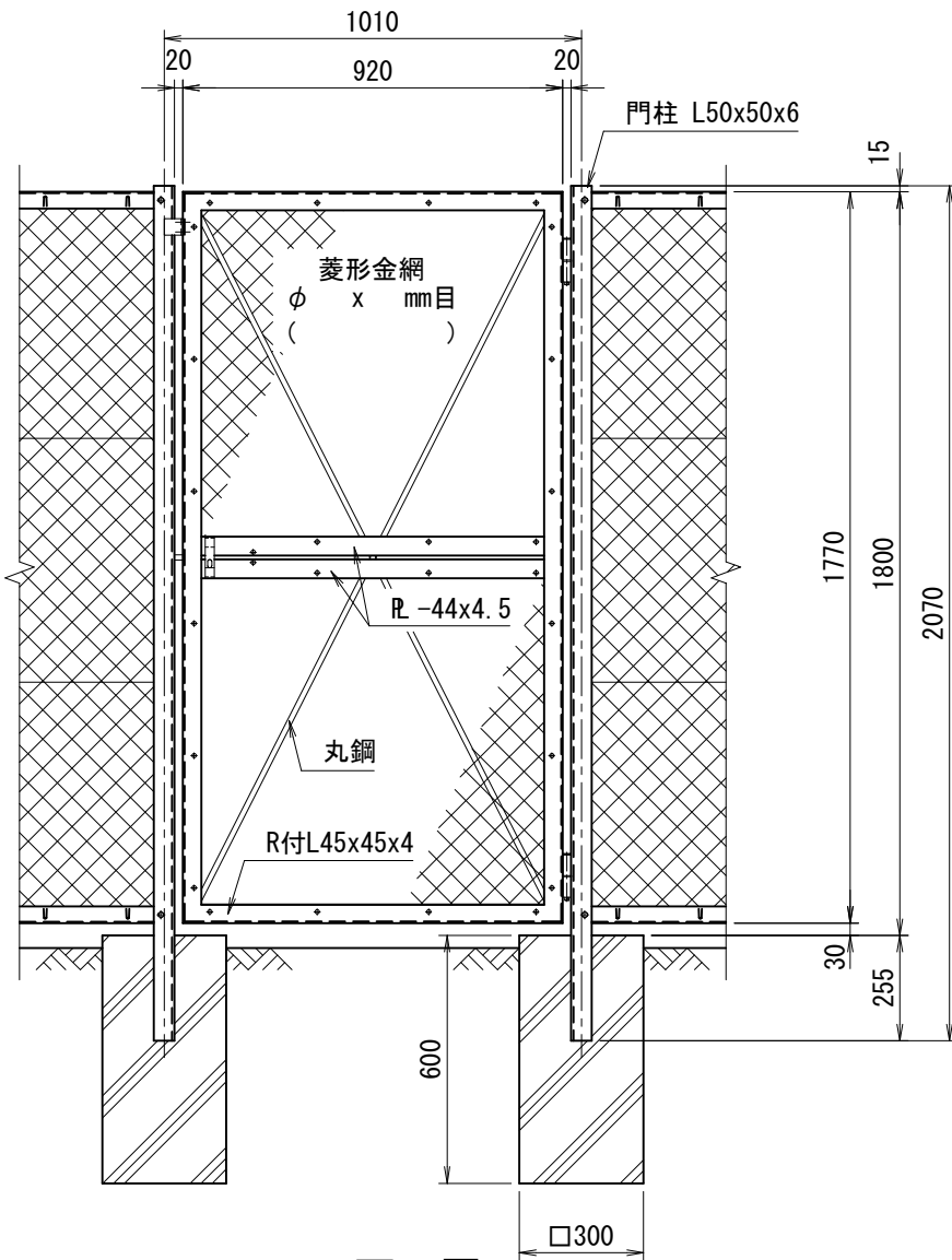
正面図 (S=1/20)
