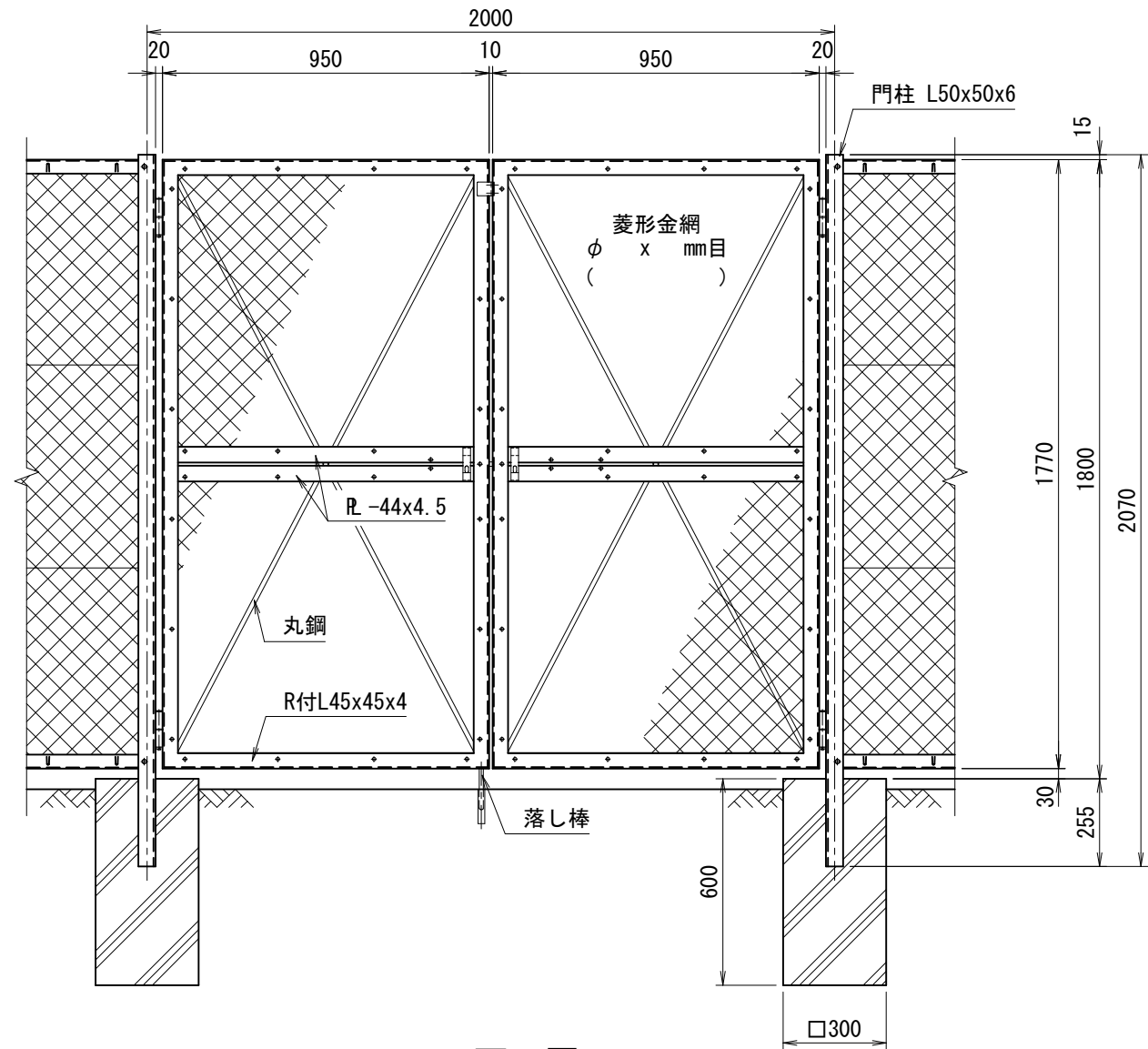
正面図 (S=1/20)
