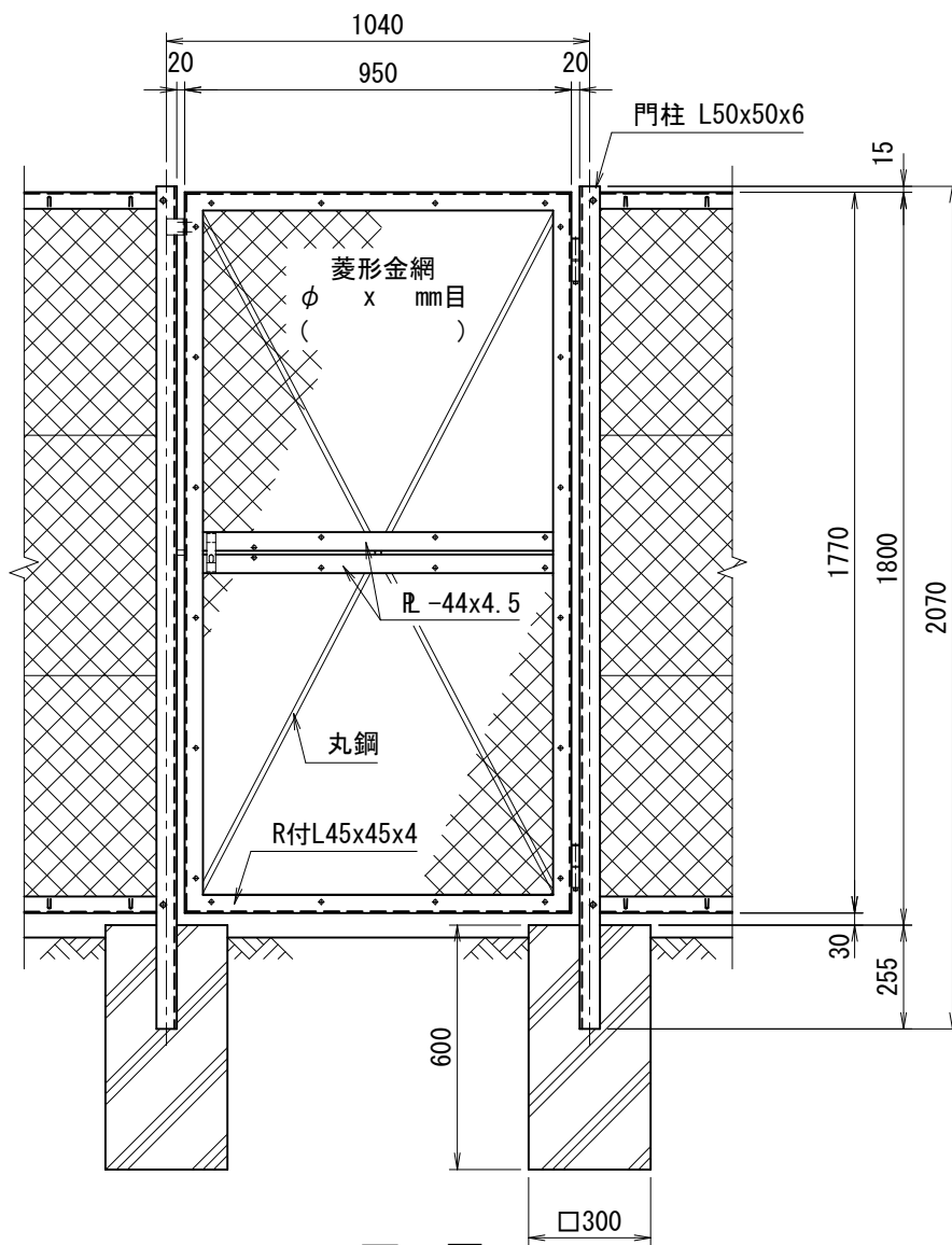
正面図 (S=1/20)
