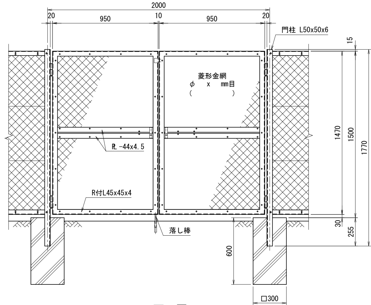
正面図 (S=1/20)
