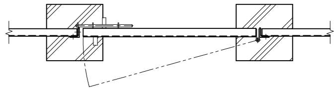
平面図 (S=1/20)
