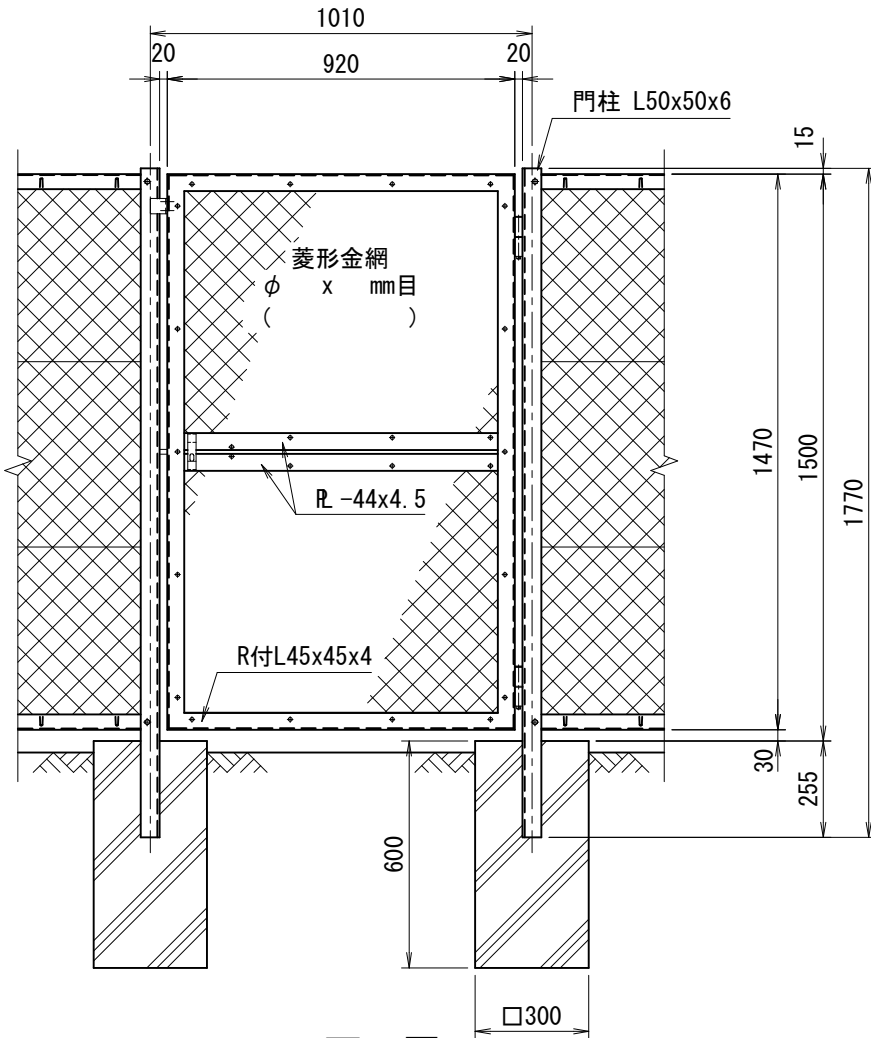
正面図 (S=1/20)
