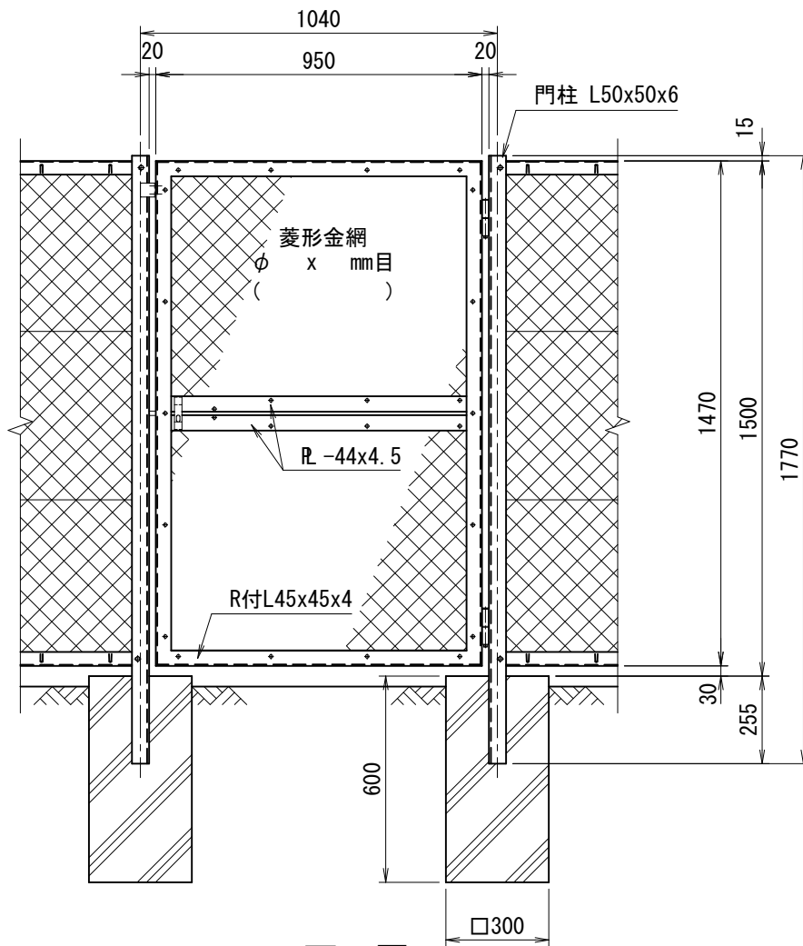
正面図 (S=1/20)
