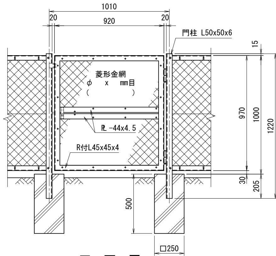
正面図 (S=1/20)
