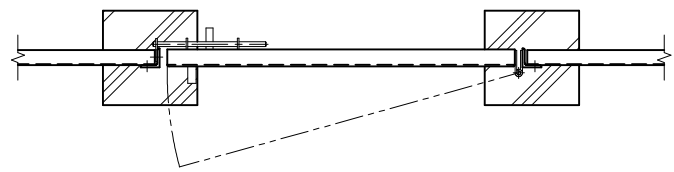
平面図 (S=1/20)
