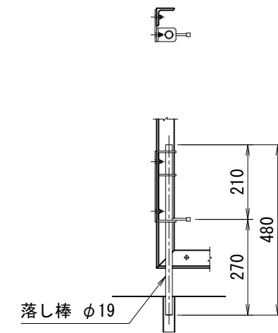
落とし棒取付詳細図
