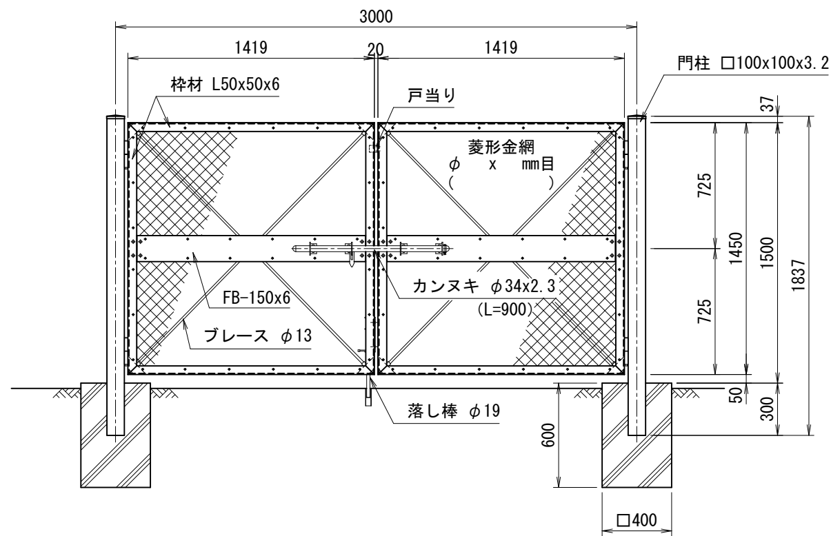
正面図 (S=1/30)
