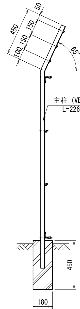
側面図 (S=1/20)
