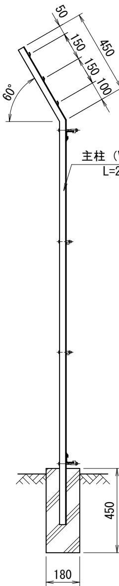
側面図 (控無) (S=1/20)
