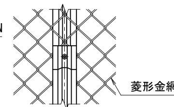
控柱取付詳細
