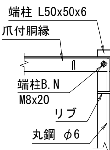
端柱取付詳細
