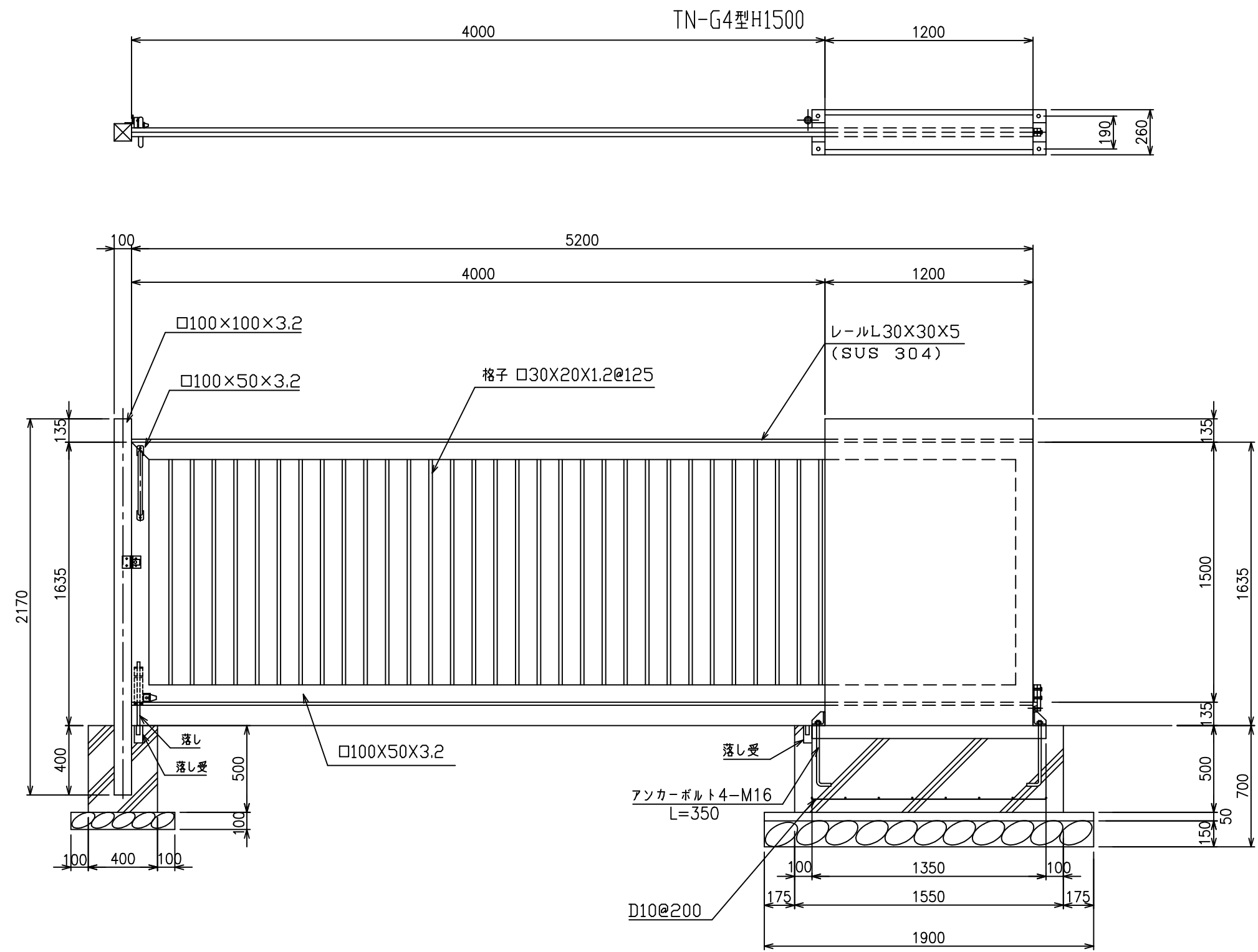
正面図 (S=1/20)
