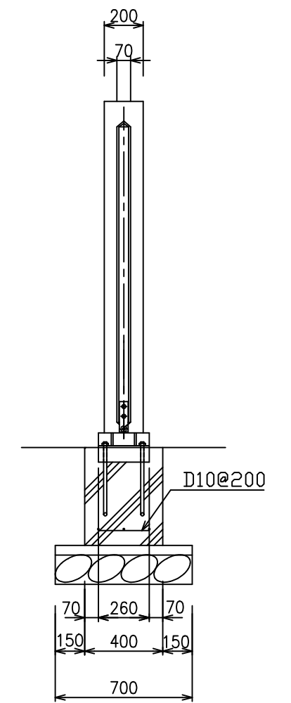
側面図 (S=1/20)
