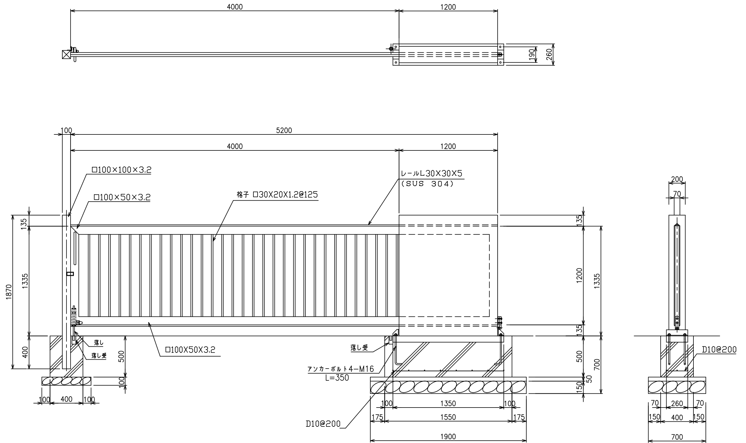
正面図 (S = 1/20)
