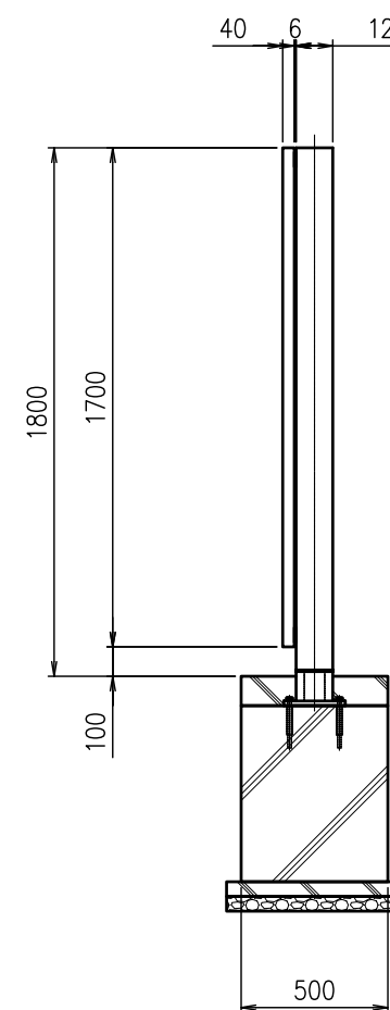
側面図
