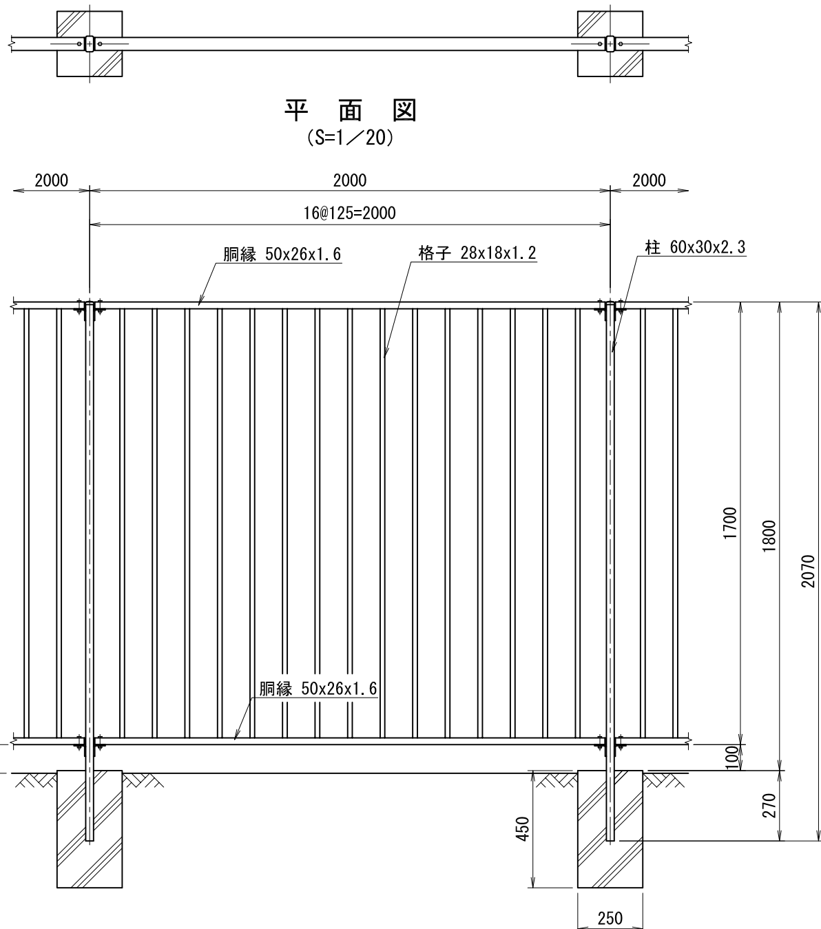
正面図 (S=1/20)
