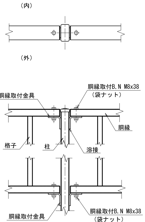
柱・胴縁取付詳細
