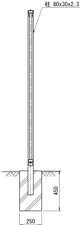
側面図 (S=1/20)
