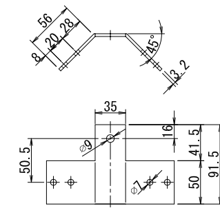
コーナープレート (隅柱部品)
