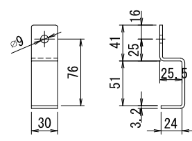
胴縁支金具
