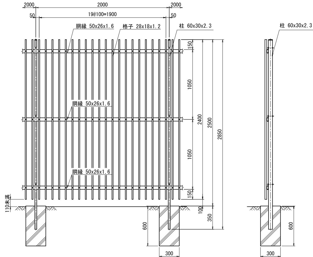
正面図 (S=1/30)
