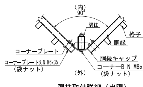
隅柱取付詳細 (出隅)
