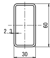
柱断面図 (S=1/2)
