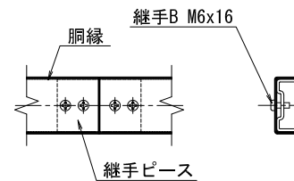
胴縁・継手取付詳細
