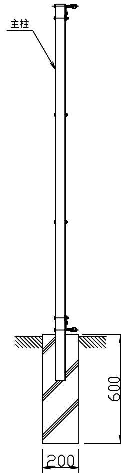
側面図 (S=1/15)
