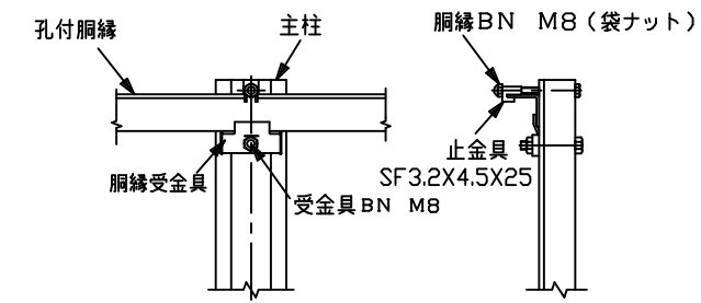
支柱・胴縁取付詳細
