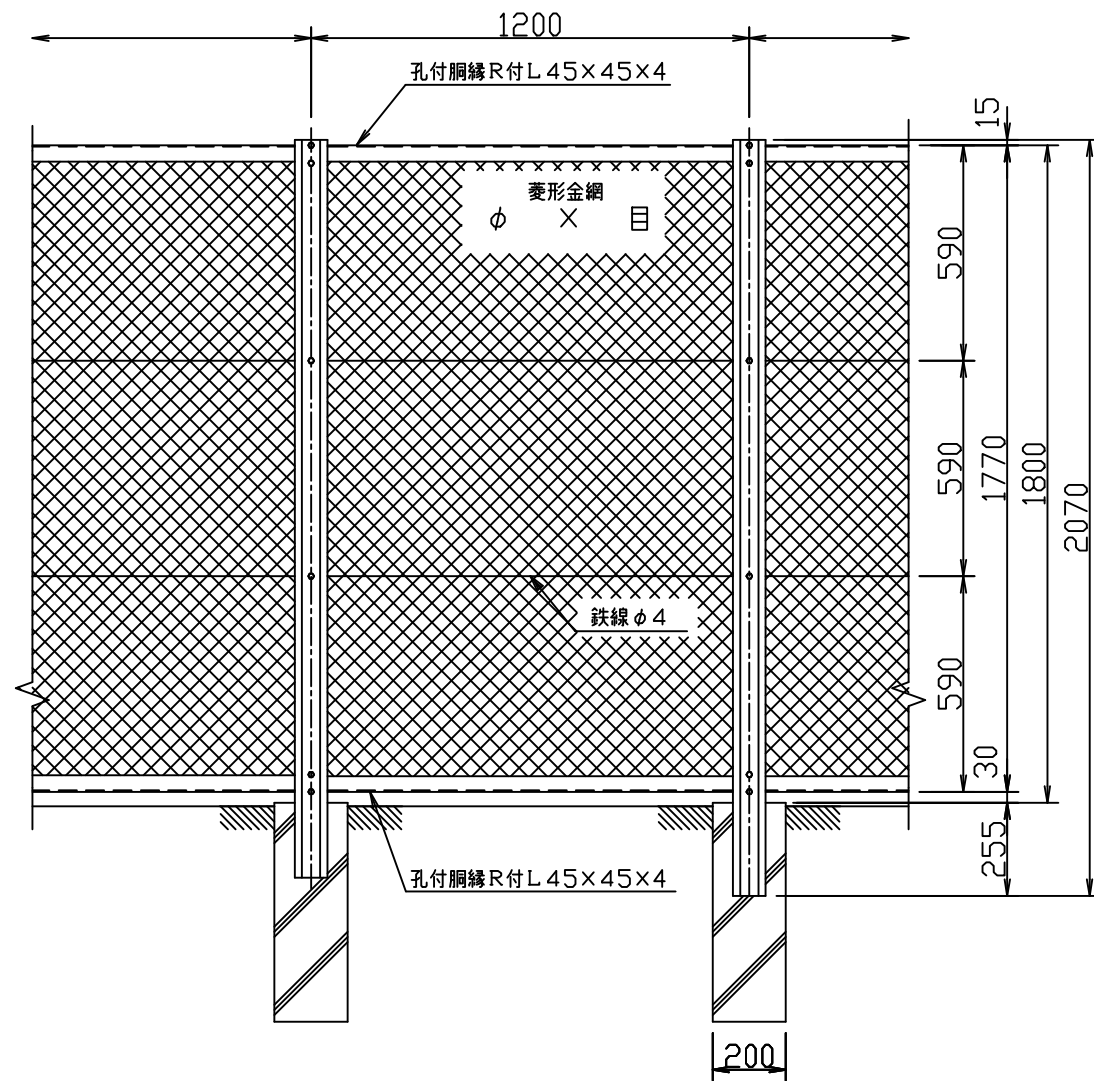
正面図 (S=1/15)
