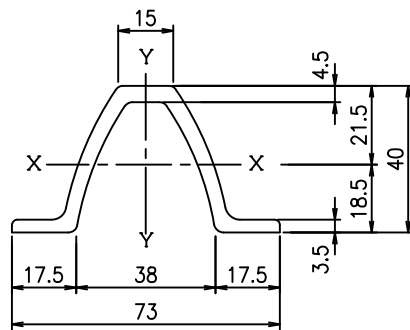
主柱断面図 (VB) (S=1/1)
