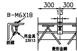
吊金具・金網取付詳細
