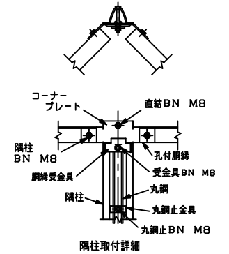
隅柱取付詳細
