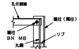
端柱 (隅柱) 取付詳細
