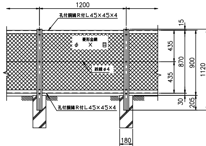
正面図 (S=1/15)
