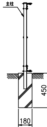
側面図 (S=1/15)
