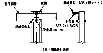
主柱・網締取付詳細
