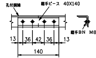
網締・継手ピース取付詳細
