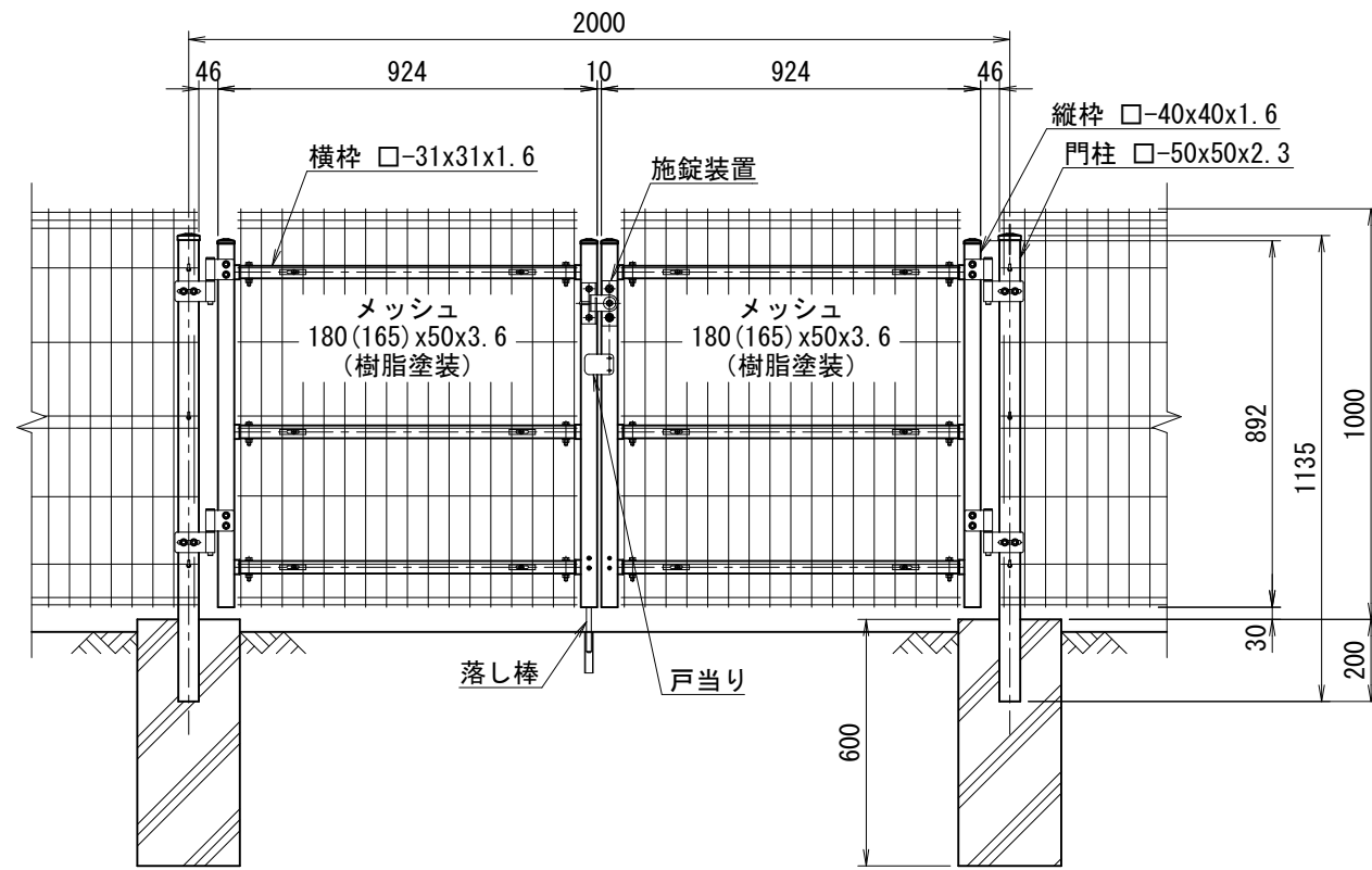
正面図 (S=1/20)
