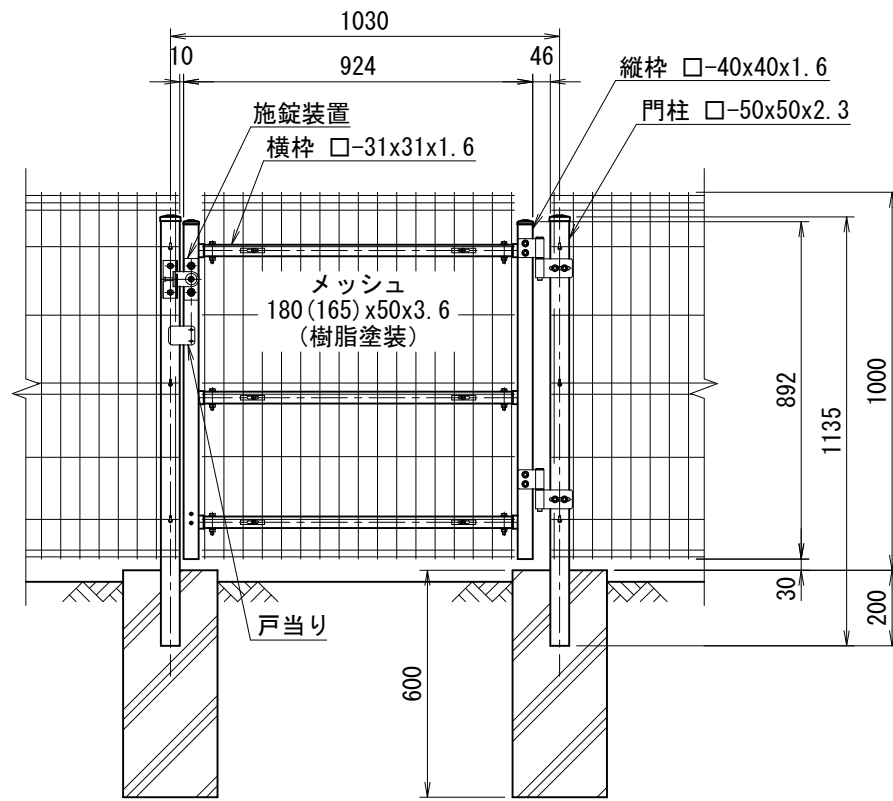
正面図 (S=1/20)
