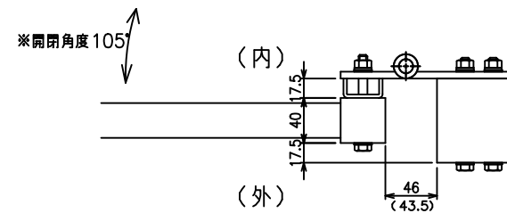
内開き丁番取付詳細図
