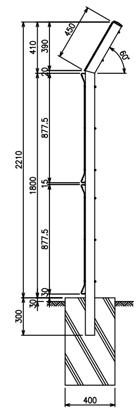
フェンス部断面図 (S=1/30)
