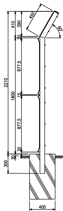
フェンス部断面図 (S=1/30)
