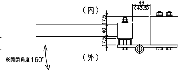
外開き丁番取付詳細図
