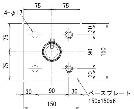
正面図 (S=1/20)
