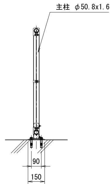
側面図 (S=1/20)
