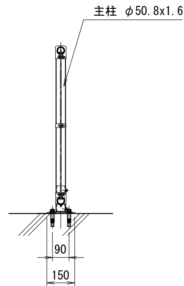
側面図 (S=1/20)
