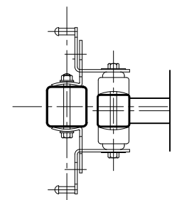
片開き施錠詳細図
