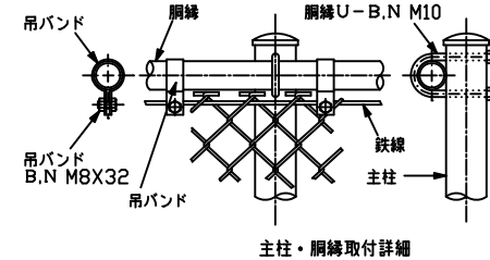
主柱・上綱取付詳細
