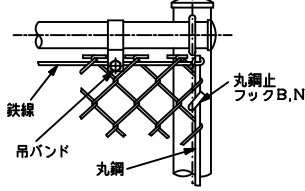
下綱・継手ベース取付詳細
