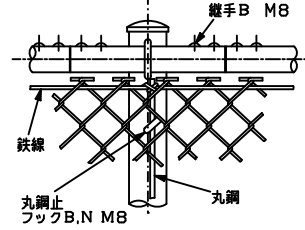
隅柱取付詳細
