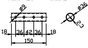
上継手ベース(寸法記号36X150)
