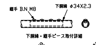
下綱・継手ベース取付詳細
