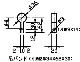
吊バンド(寸法記号34X62X30)
