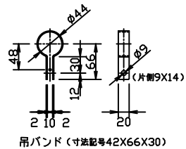
吊バンド(寸法記号42X66X30)
