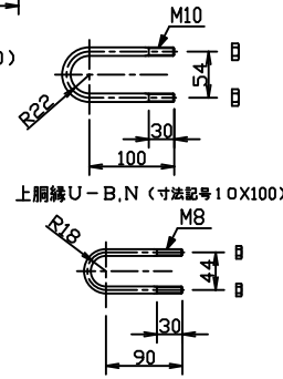
下綱U-B,N(寸法記号8X90)
