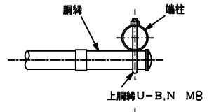
上綱・継手ベース取付詳細
