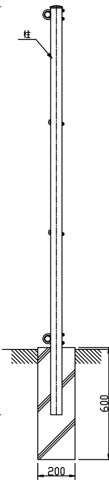
側面図 (S=1/10)
