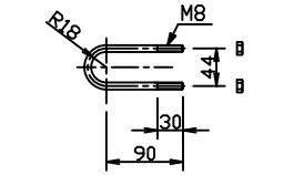
下綱U-B,N(寸法記号8X90)
