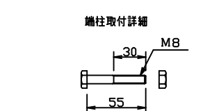
上継手B(寸法記号8X55)
