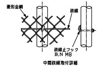
中間鉄線取付詳細
