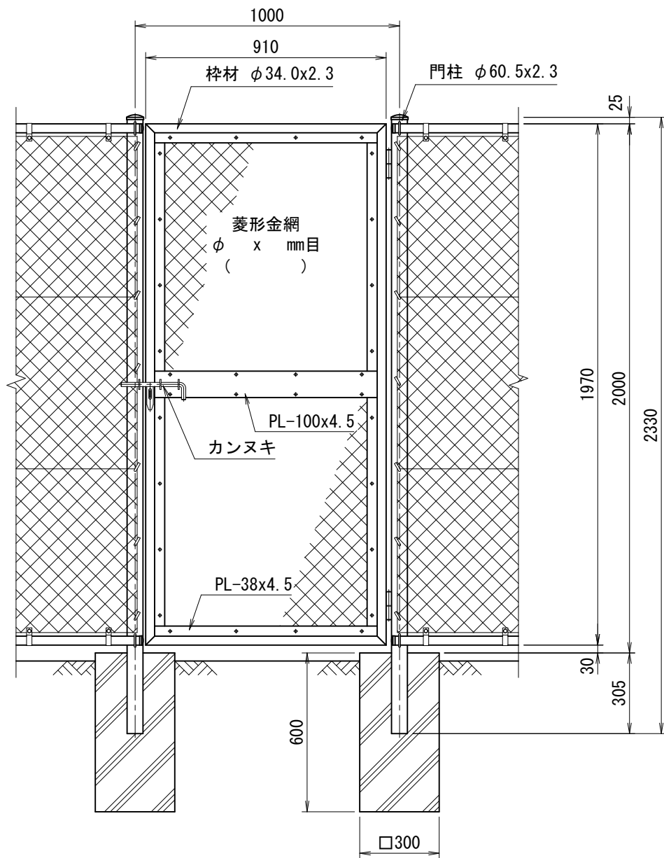
正面図 (S=1/20)
