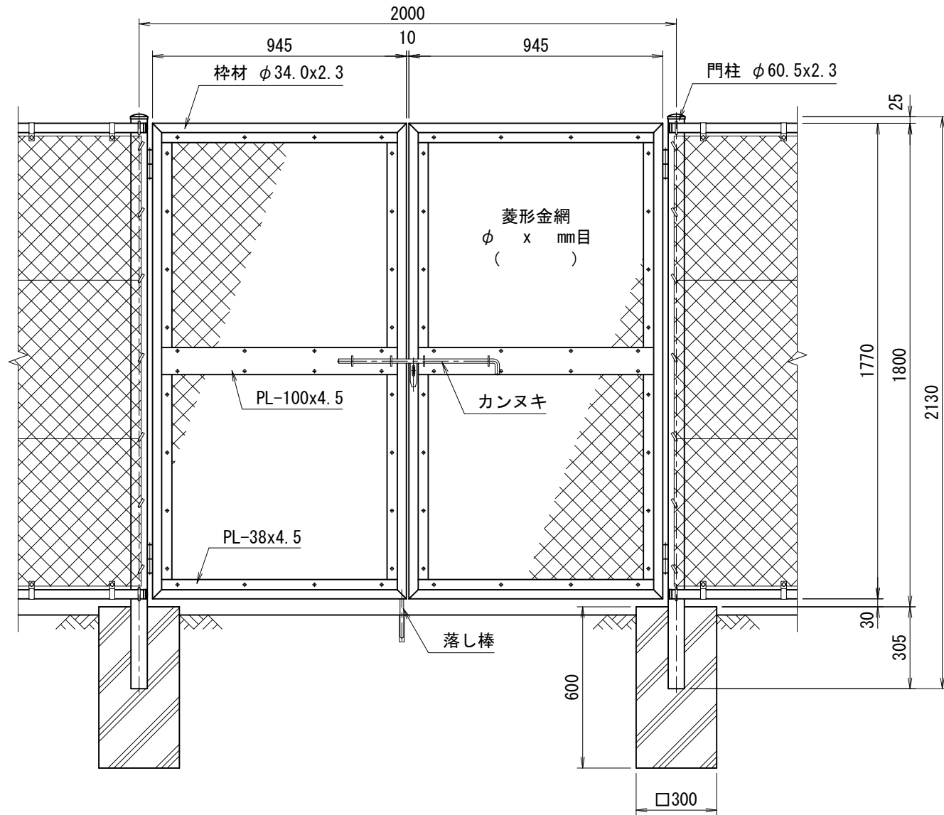
正面図 (S=1/20)
