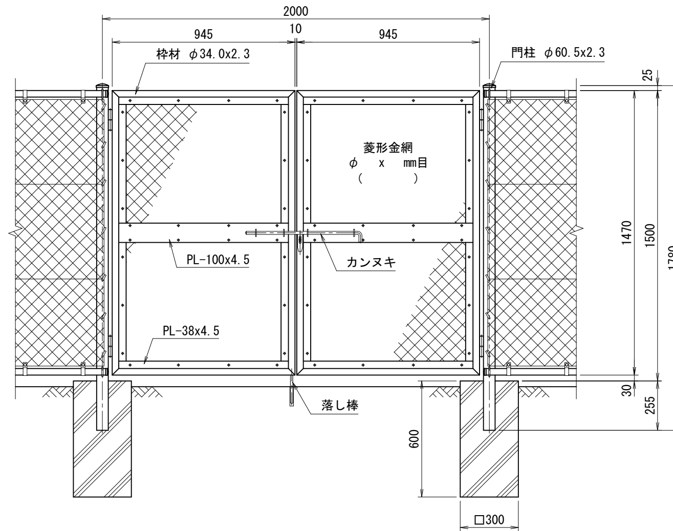
正面図 (S=1/20)
