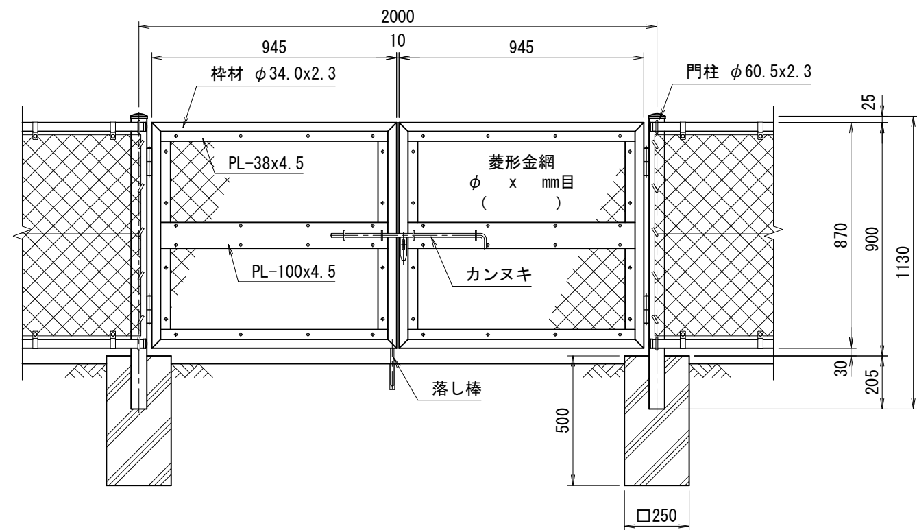
正面図 (S=1/20)
