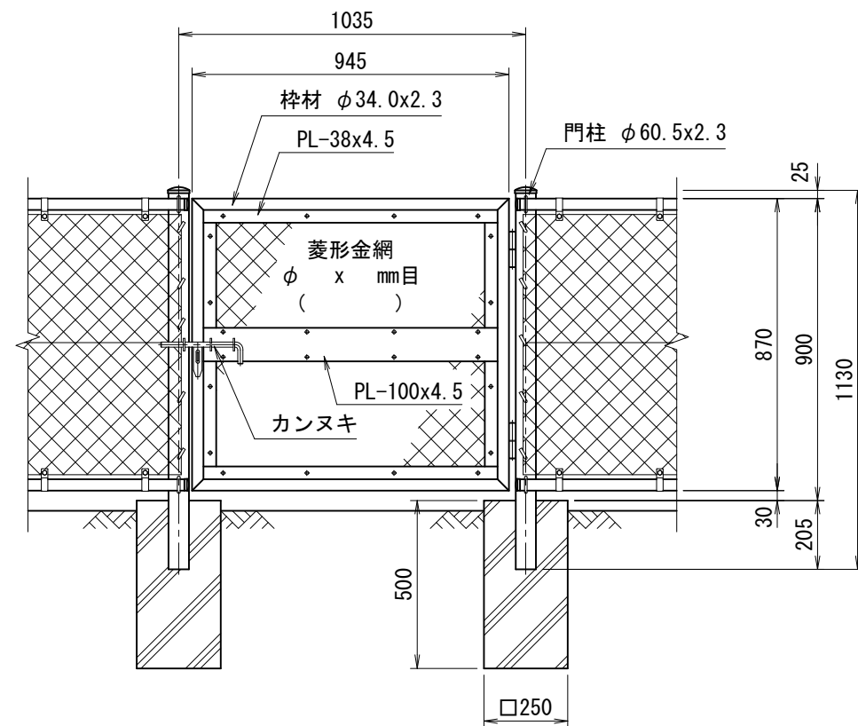
正面図 (S=1/20)
