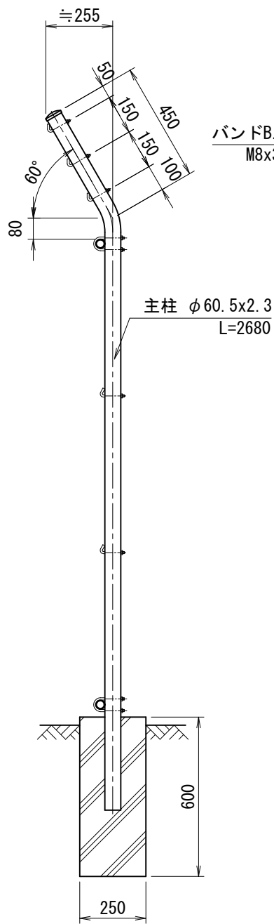
側面図 (S=1/20)
