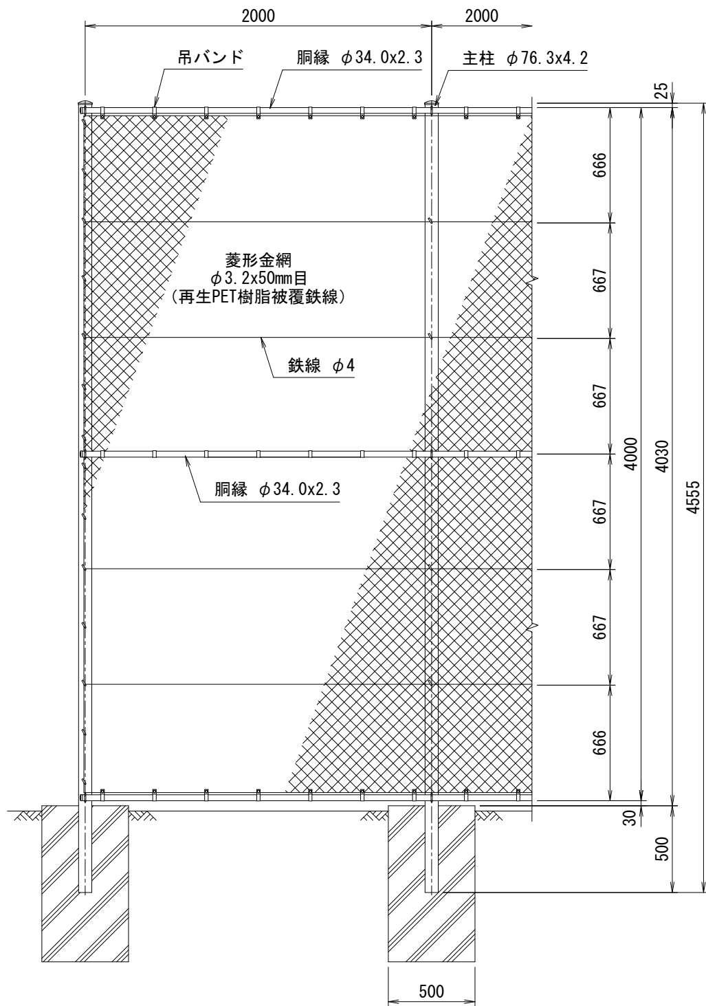
正面図 (S=1/30)
