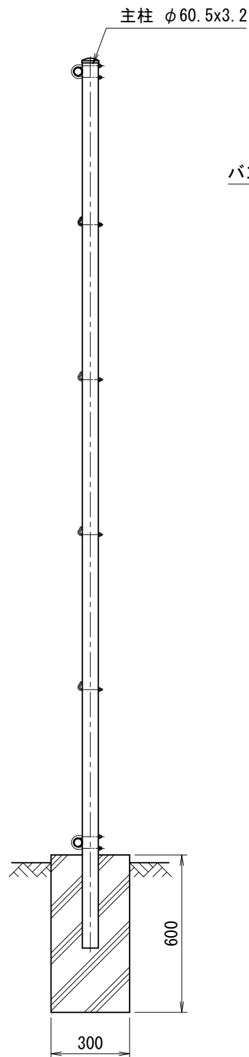
側面図 (S=1/20)
