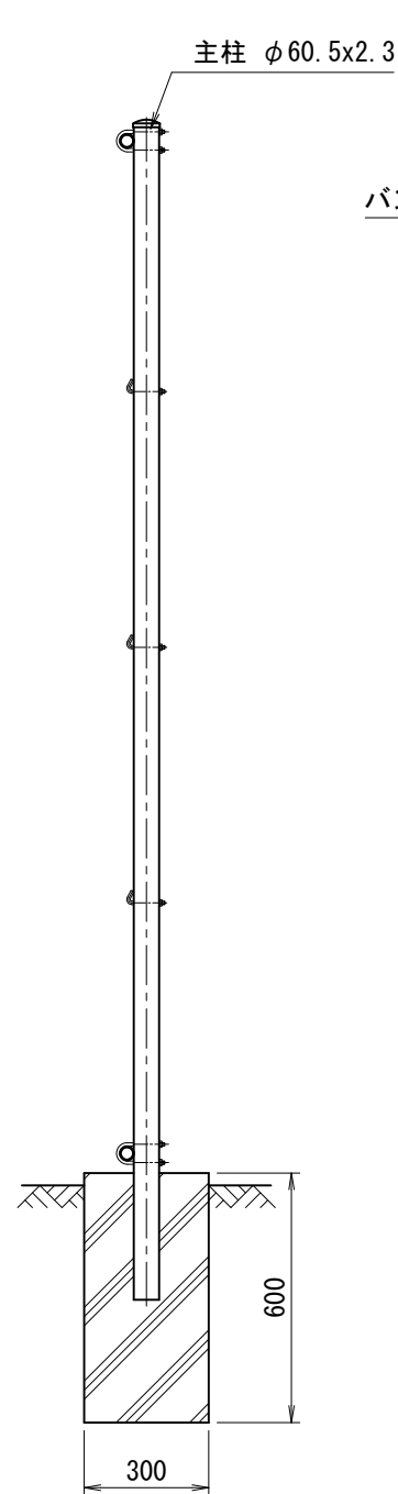
側面図 (S=1/20)
