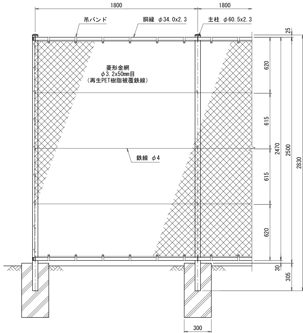
正面図 (S=1/20)
