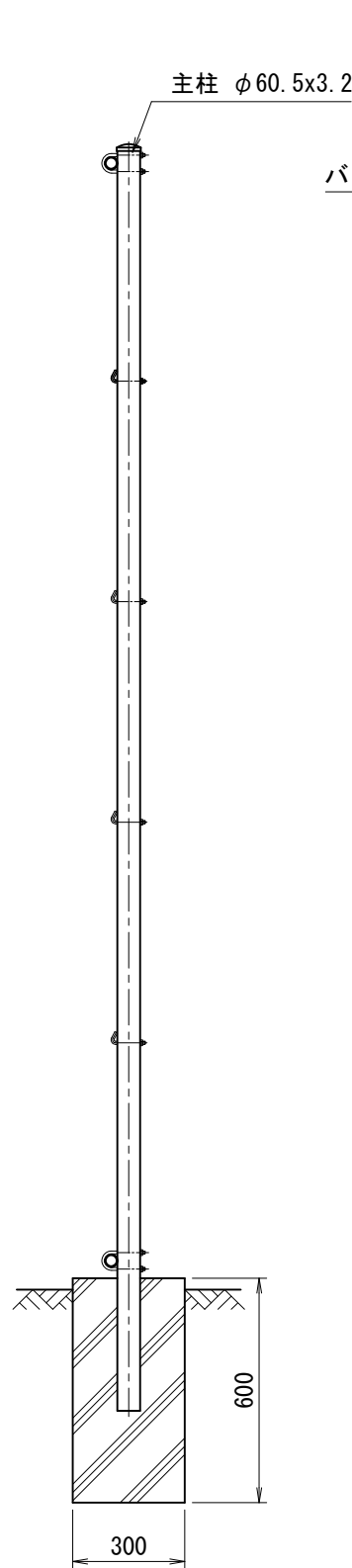
側面図 (S=1/20)
