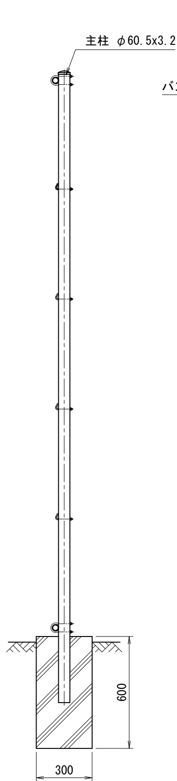
側面図 (S=1/20)
