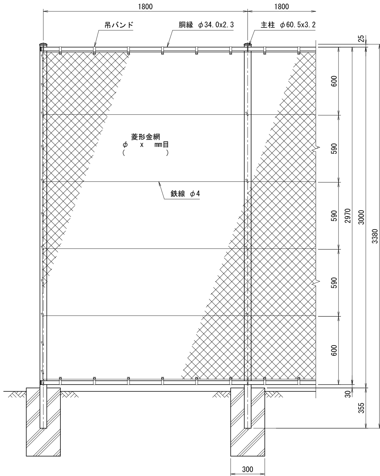
正面図 (S=1/20)
