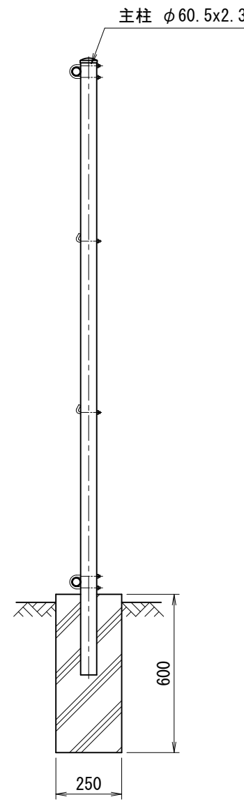
側面図 (S=1/20)
