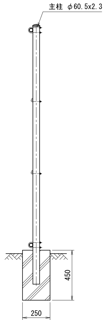
側面図 (S=1/20)
