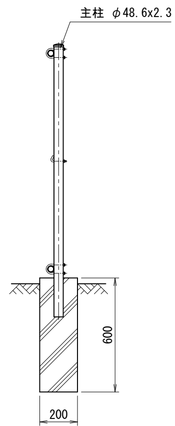
側面図 (S=1/20)
