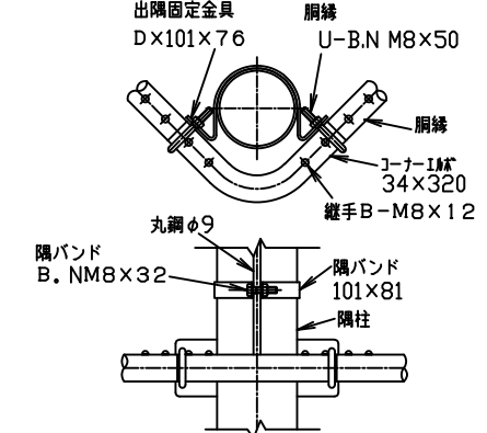
出隅下胴縁取付詳細
