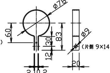
吊バンド (寸法記号 76×83×30)
