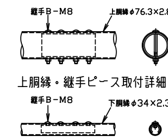
上胴縁・継手ピース取付詳細
