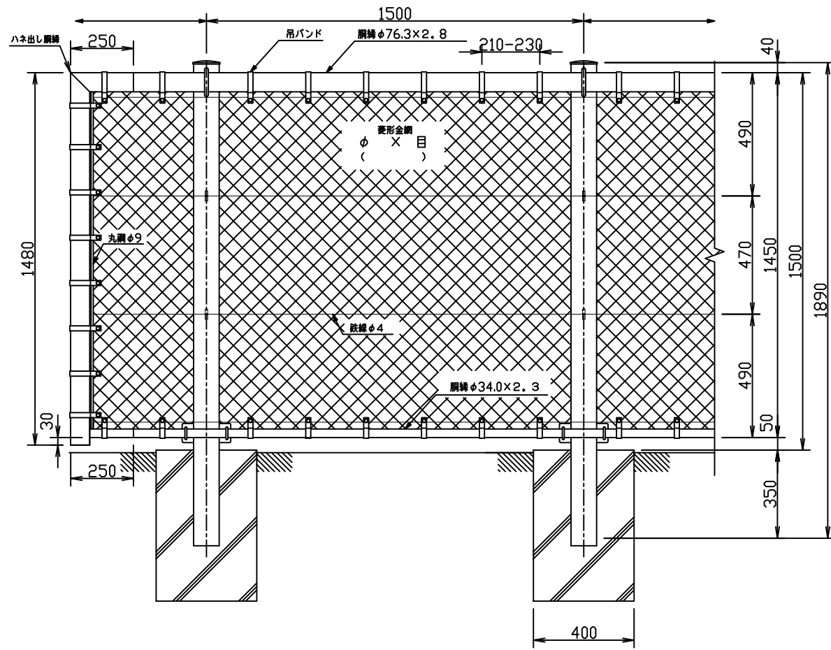
正面図 (S=1/15)
