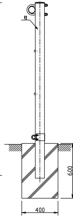
側面図 (S=1/15)
