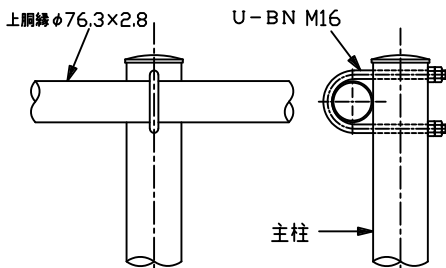
柱・上胴縁取付詳細
