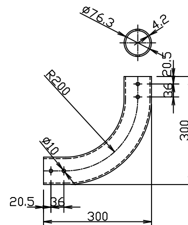
上コーナーエルボ (寸法記号 48×200C)
