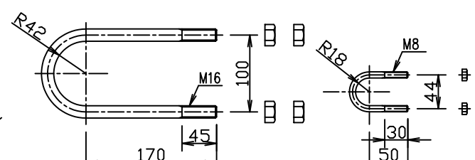
胴縁固定金具 (寸法記号 101×196)
