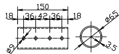
下胴縁・継手ピース取付詳細
