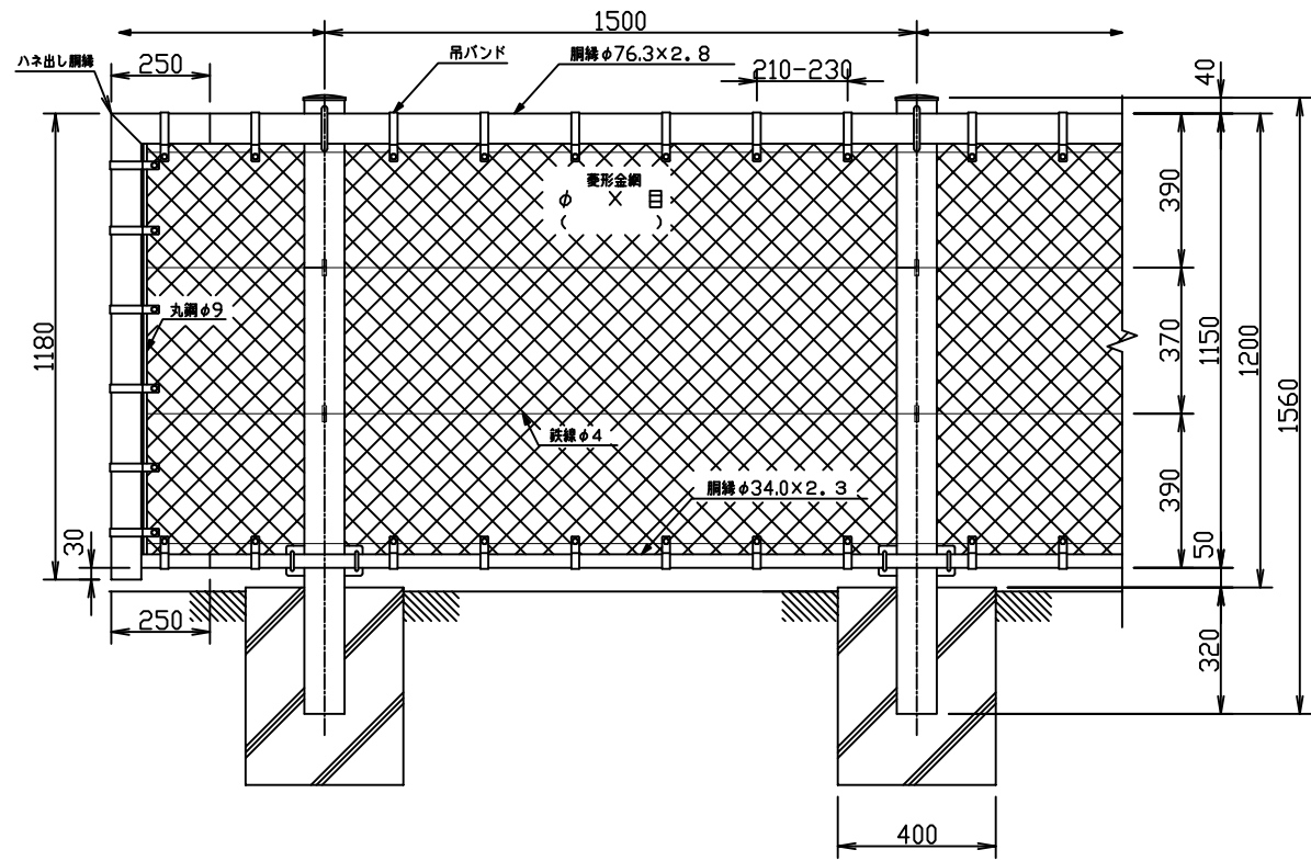
正面図 (S=1/15)
