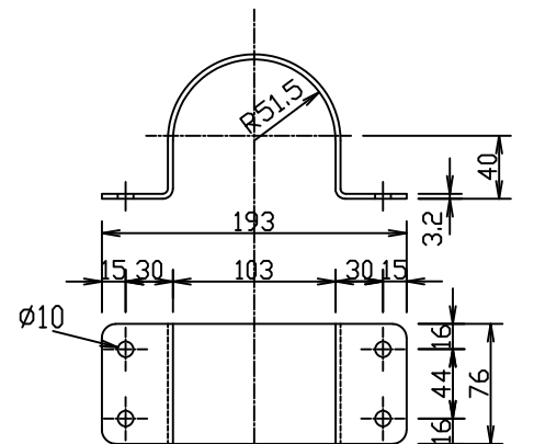
胴縁固定金具 (寸法記号 101×196)
