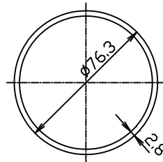
上胴縁断面図 (S=1/2)
