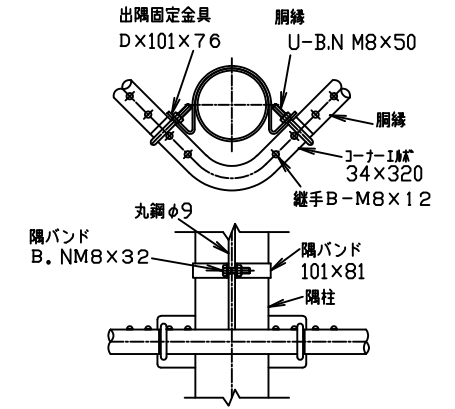
出隅下胴縁取付詳細
