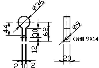
吊バンド (寸法記号 34×62×30)
