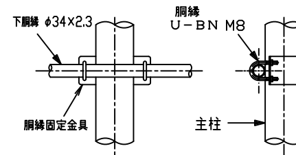
柱・下胴縁取付詳細
