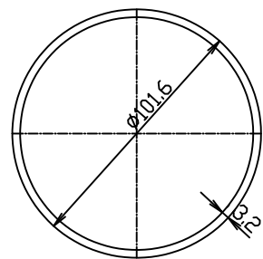
柱断面図 (S=1/2)
