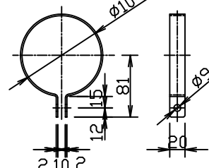
隅バンド (寸法記号 101×81)
