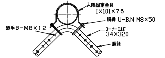
入隅下胴縁取付詳細
