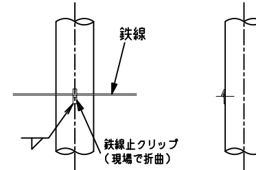
中間鉄線取付詳細
