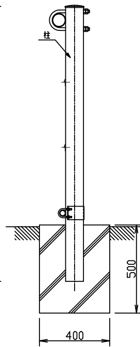
側面図 (S=1/15)
