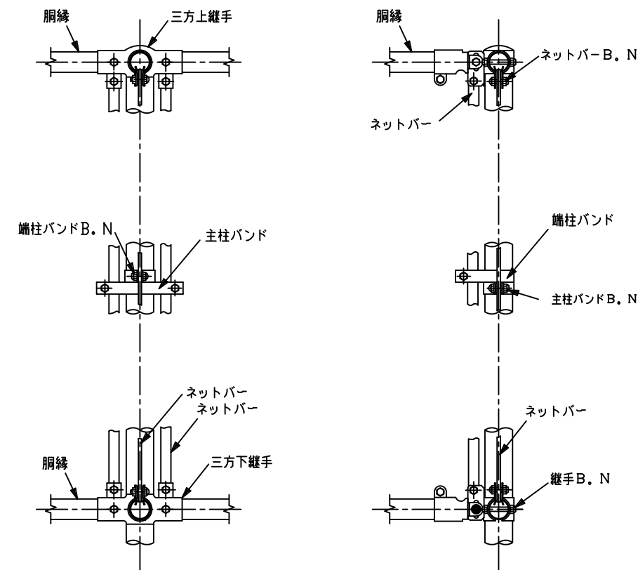
三方部取付詳細
